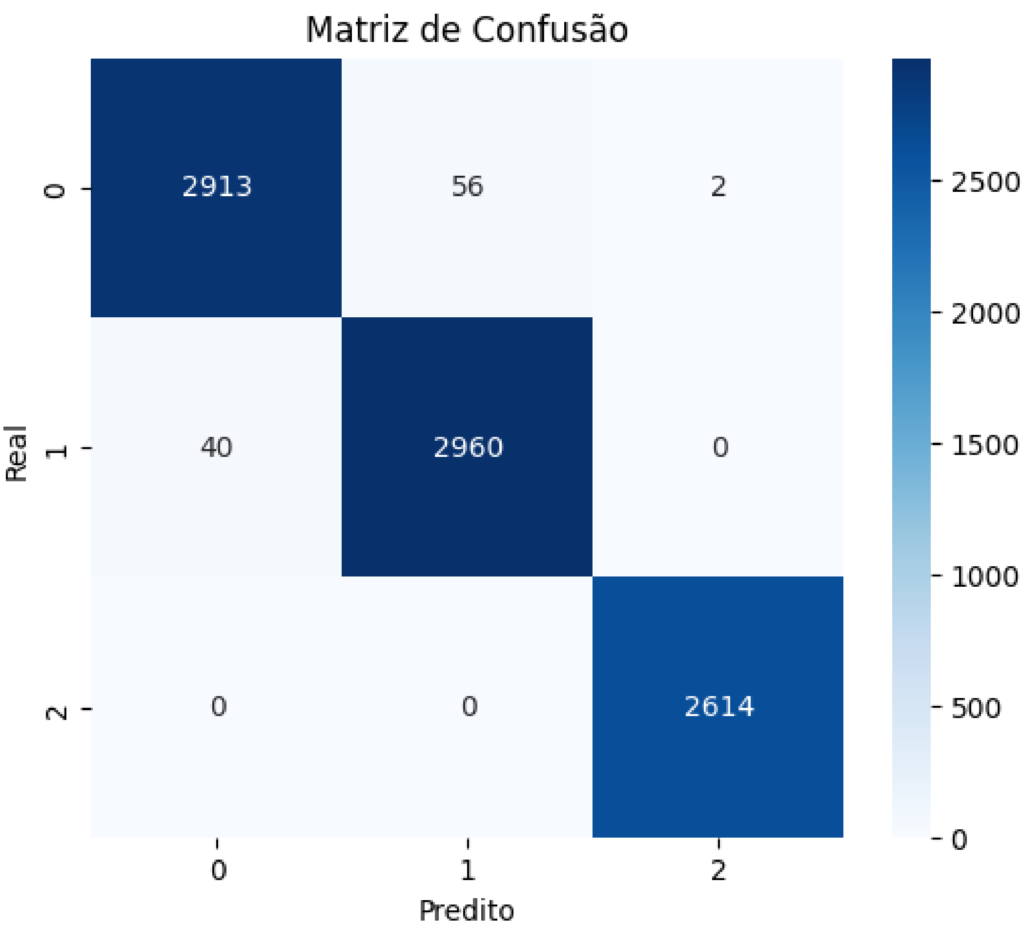
Figura 3: Matriz de confusão do modelo Random Forest
